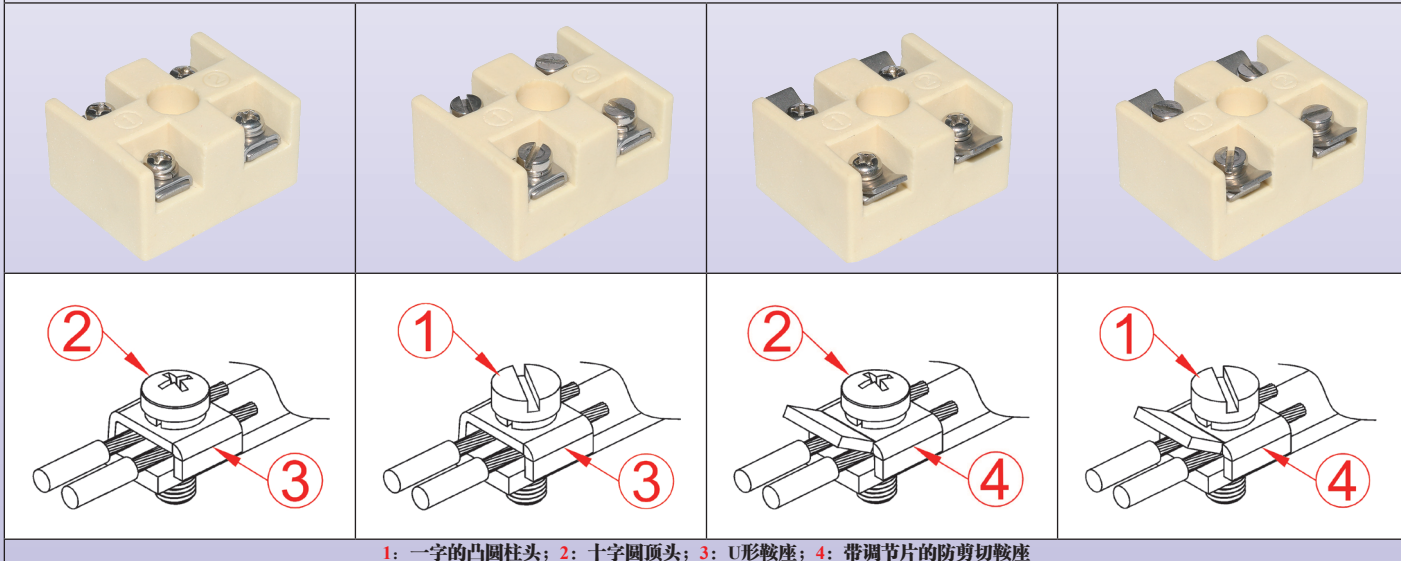
1: 一字的凸圆柱头; 2: 十字圆顶头; 3: U形鞍座; 4: 带调节片的防剪切鞍座
